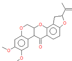
Rotenone
